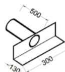
Desagüe lateral circular PVC
