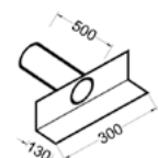
Desagüe lateral circular TPO
