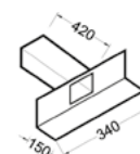
Desagüe lateral rectangular PVC
